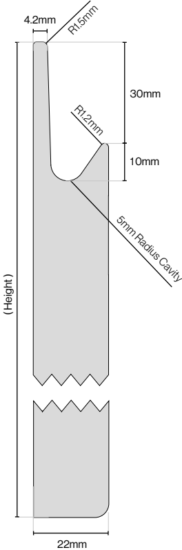
Luzzi Door Cross Section
