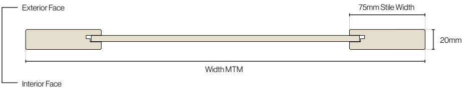
Monroe Door Cross Section
