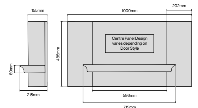
Classic Canopy 1000mm (W) x 215mm (D) x 485mm (H)
