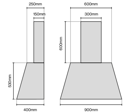
Chimney Canopy 900mm (W) x 400mm (D) x 1130mm (H)
