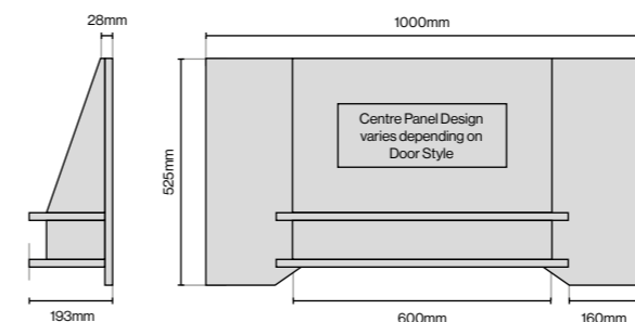
Modern Canopy 1000mm (L) x 193mm (D) x 525mm (H)
