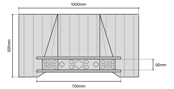
Traditional Canopy* 1000mm (L) x 193mm (D) x 525mm (H)
